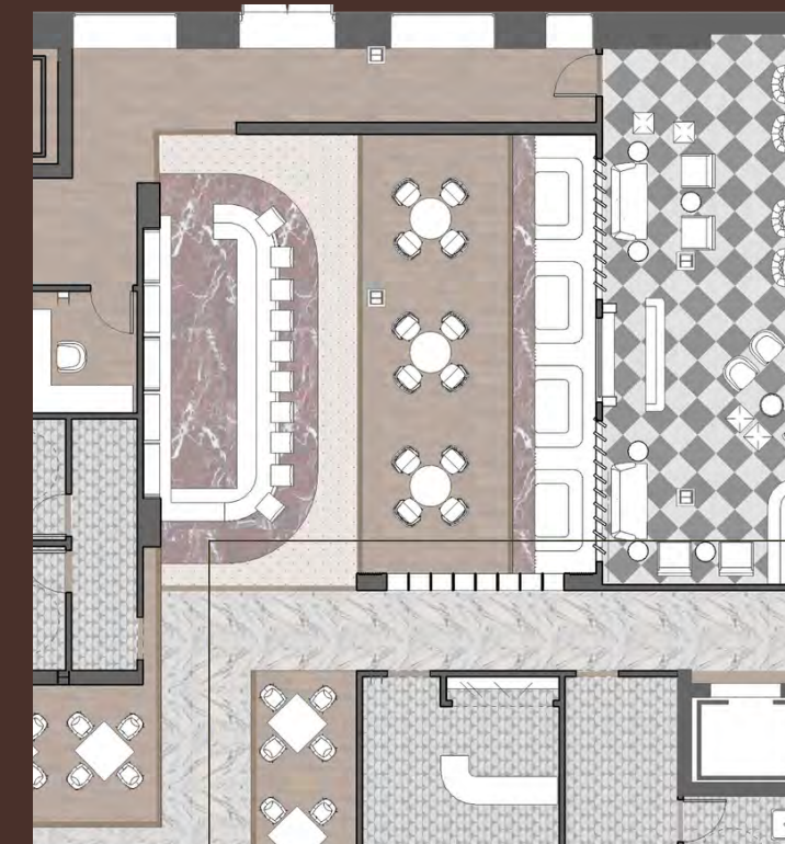
BAR PLAN
